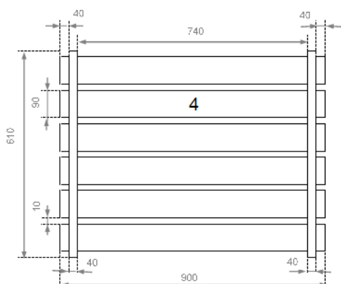
Plan de la trappe inférieure
